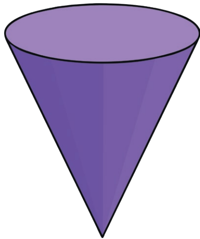
cone
