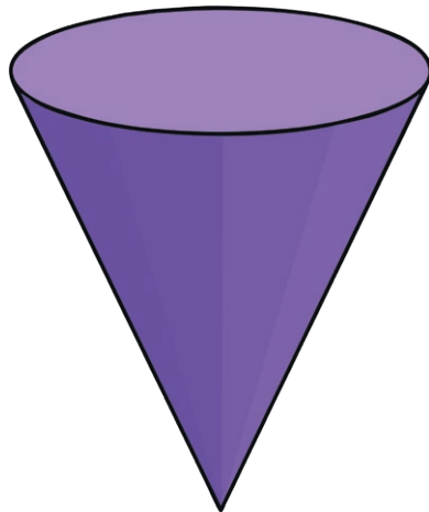
cone
