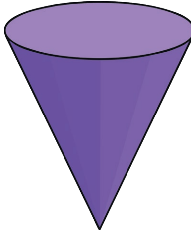
cone
