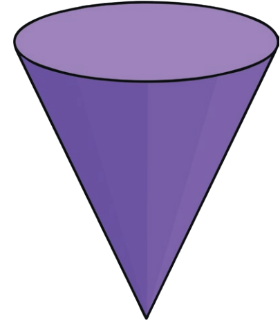
cone
