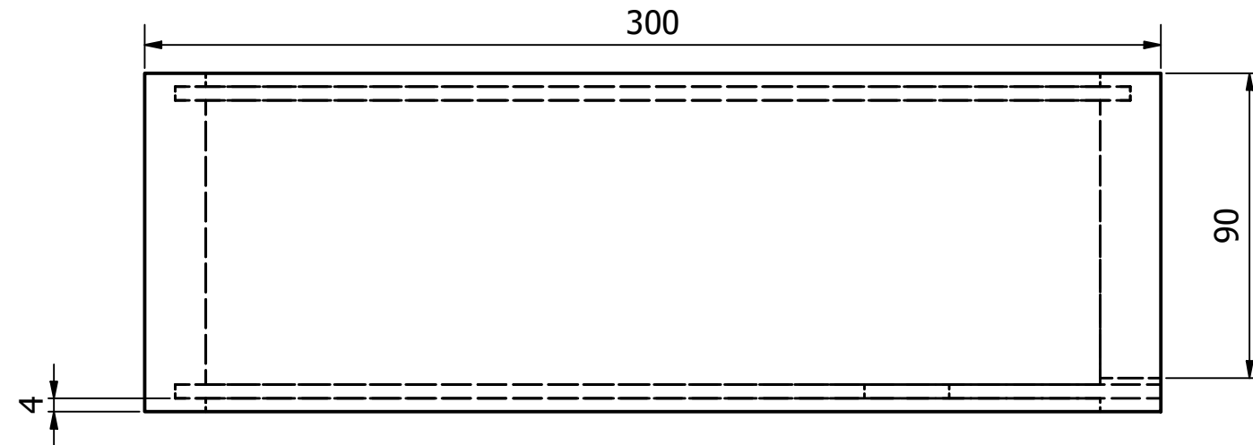
PLAN ( 1 : 2 )
